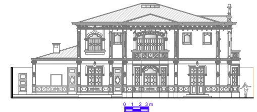
Elevação 04
