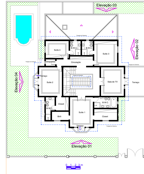
Superior
