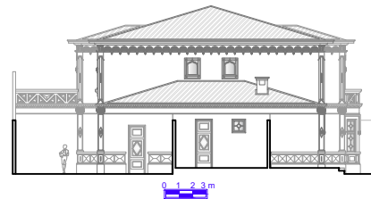
Elevação 03
