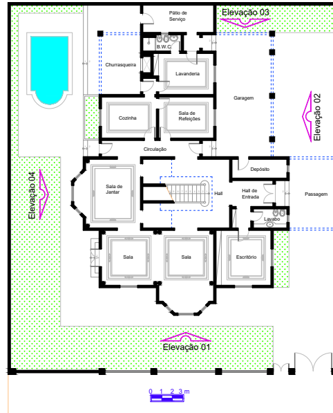
Térreo
