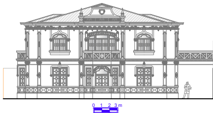
Elevação 01
